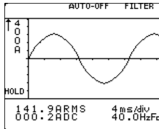
Oscilloscope Display
